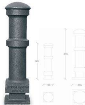
▲ BARCELONA Mod. C-42 Mod. C-42P
