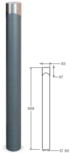
▲ DUNA Mod. C-525
