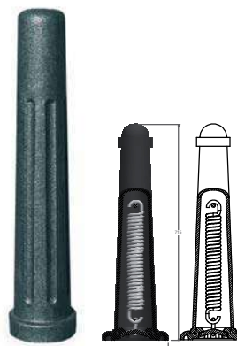
▲ FLEXIPILONA PALMA DE MALLORCA / SANT FELIU Mod. C-45PF Mod. C-41PF
